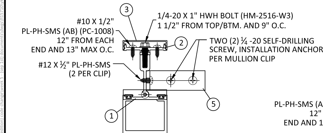
B 2 HORIZONTAL SECTION METAL STUD MULLION CLIP
